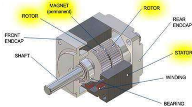
Fig 5 Stepper motor (Odhiambo, 2023)
